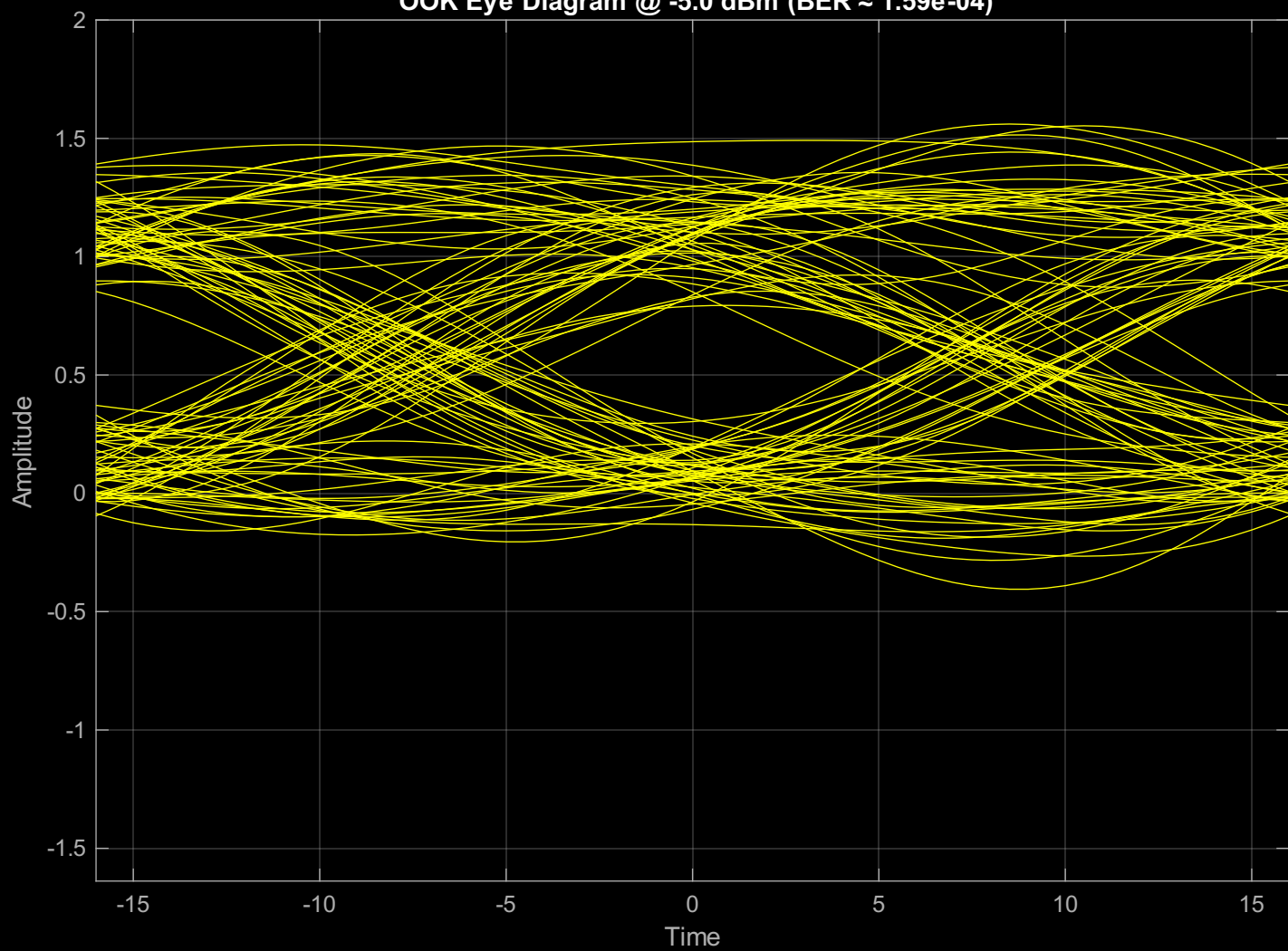
OOK Eye Diagram @ -5.0 dBm (BER \approx 1.59\text{e-}04 )
